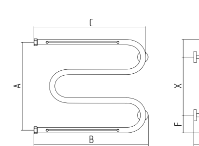
М-образный 500×650 + 2 полки **-0008-5065
