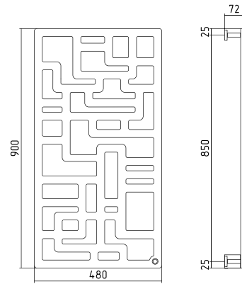
Космополит-1 900x480 **-0861-9048 Мощность: 195 W
