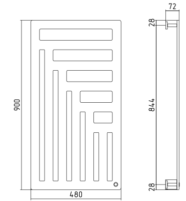
Космополит-5 900x480 **-0865-9048 Мощность: 225 W
