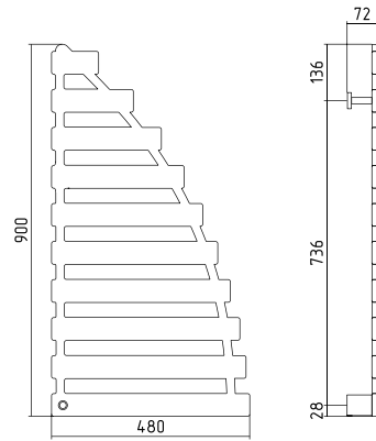
Космополит-3 900x480 **-0863-9048 Мощность: 225 W
