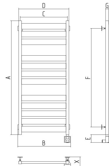
Центурион (скрытое подключение)
