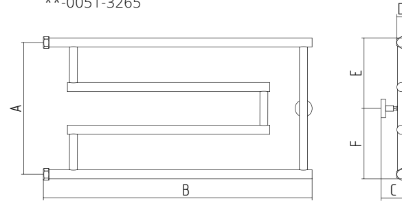
High-Tech model «G» **-0051-3265
