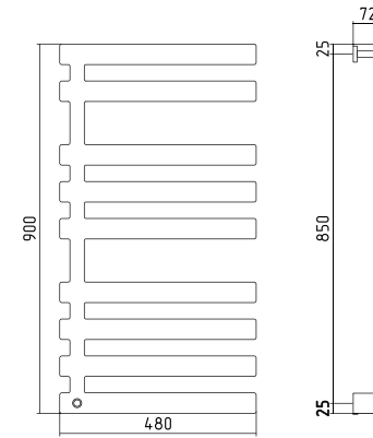
Космополит-7 900x480 **-0867-9048 Мощность: 195 W
