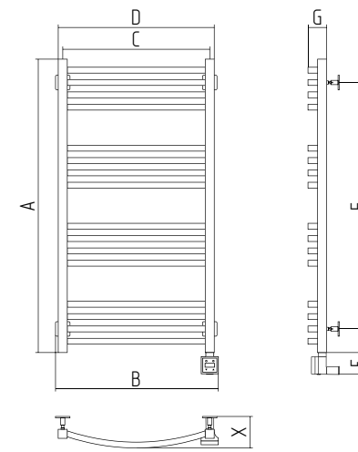
Аркус (скрытое подключение)
