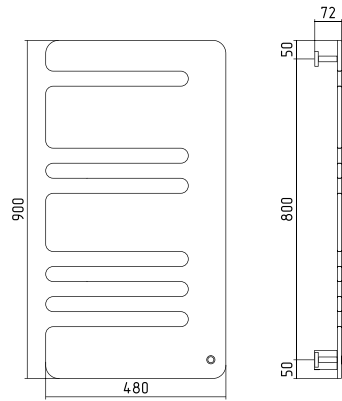
Космополит-2 900x480 **-0862-9048 Мощность: 225 W
